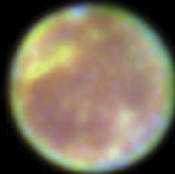
Ganymede
