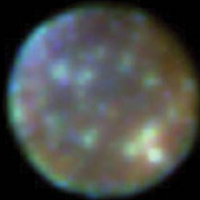
Callisto
