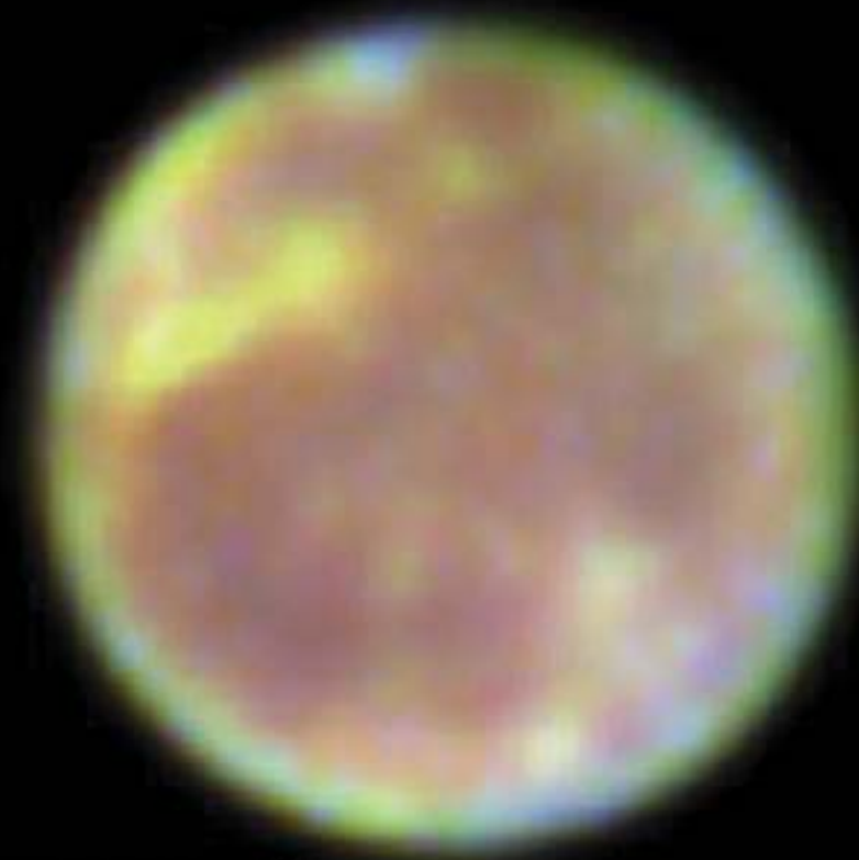
Ganymede
